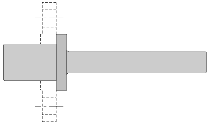
VAN STONE THERMOWELL
